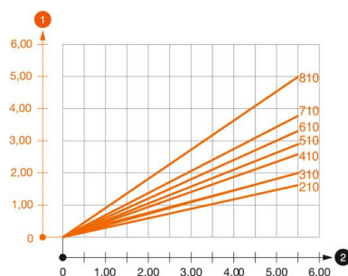
Diagramma di carico mensola tipo AS 55
