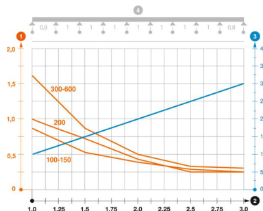
Diagramma di carico passerella grigliata tipo GRM 105
