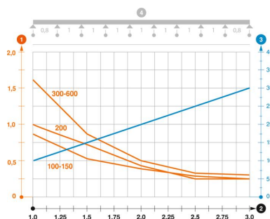
Diagramma di carico passerella grigliata tipo GRM 105
